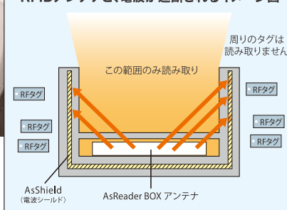
RFIDアンテナと、電波が遮断されるイメージ図
