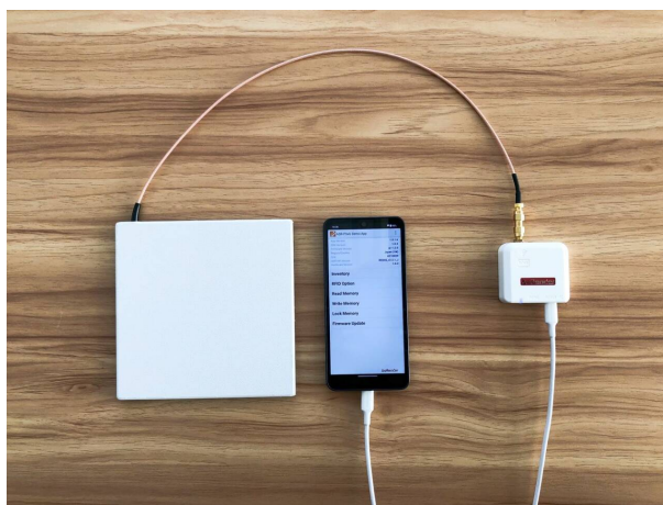
図 4-3 Android 端末の接続（方法 2）
