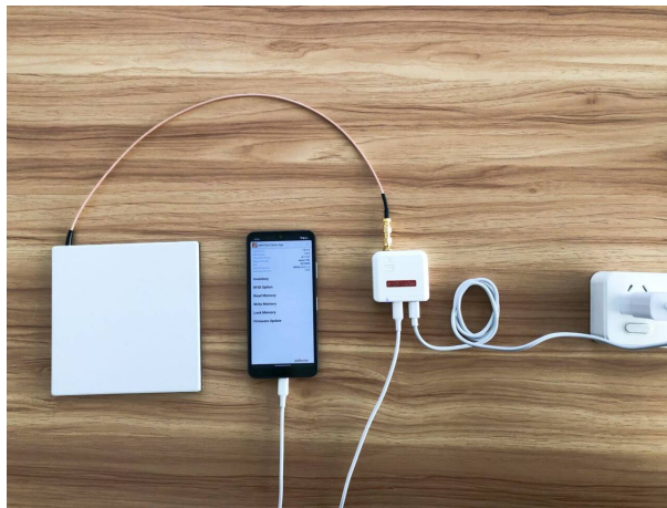
図 4-1 Android 端末の接続（方法 1）
