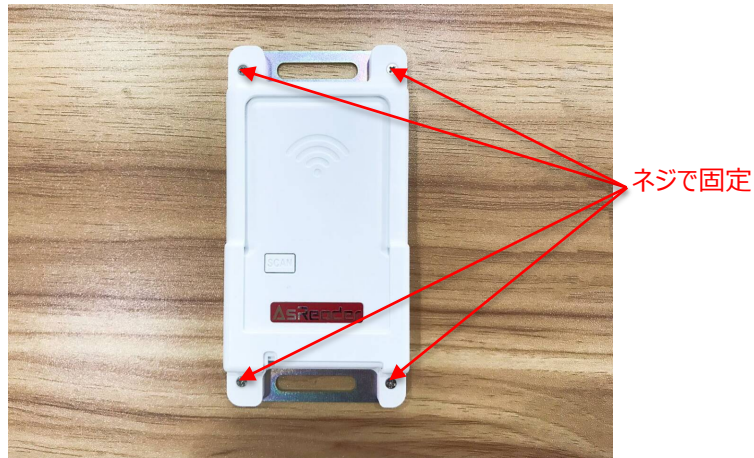
図 5-2 ASR-P35U を取り付け用フレームで挟みこんだ状態
