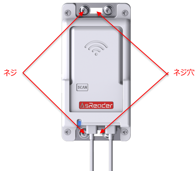
図 5-3 固定方法①
