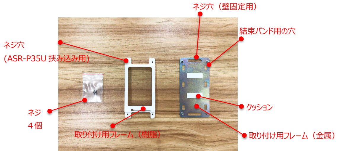
図 5.1 固定用同梱物
