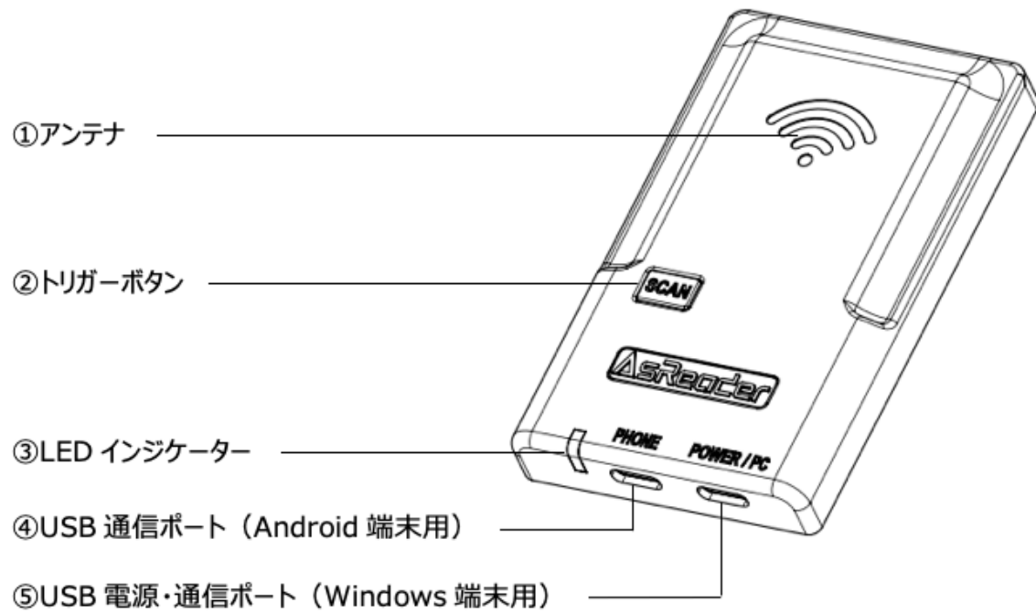
図 1-3-1 外観(正面)
